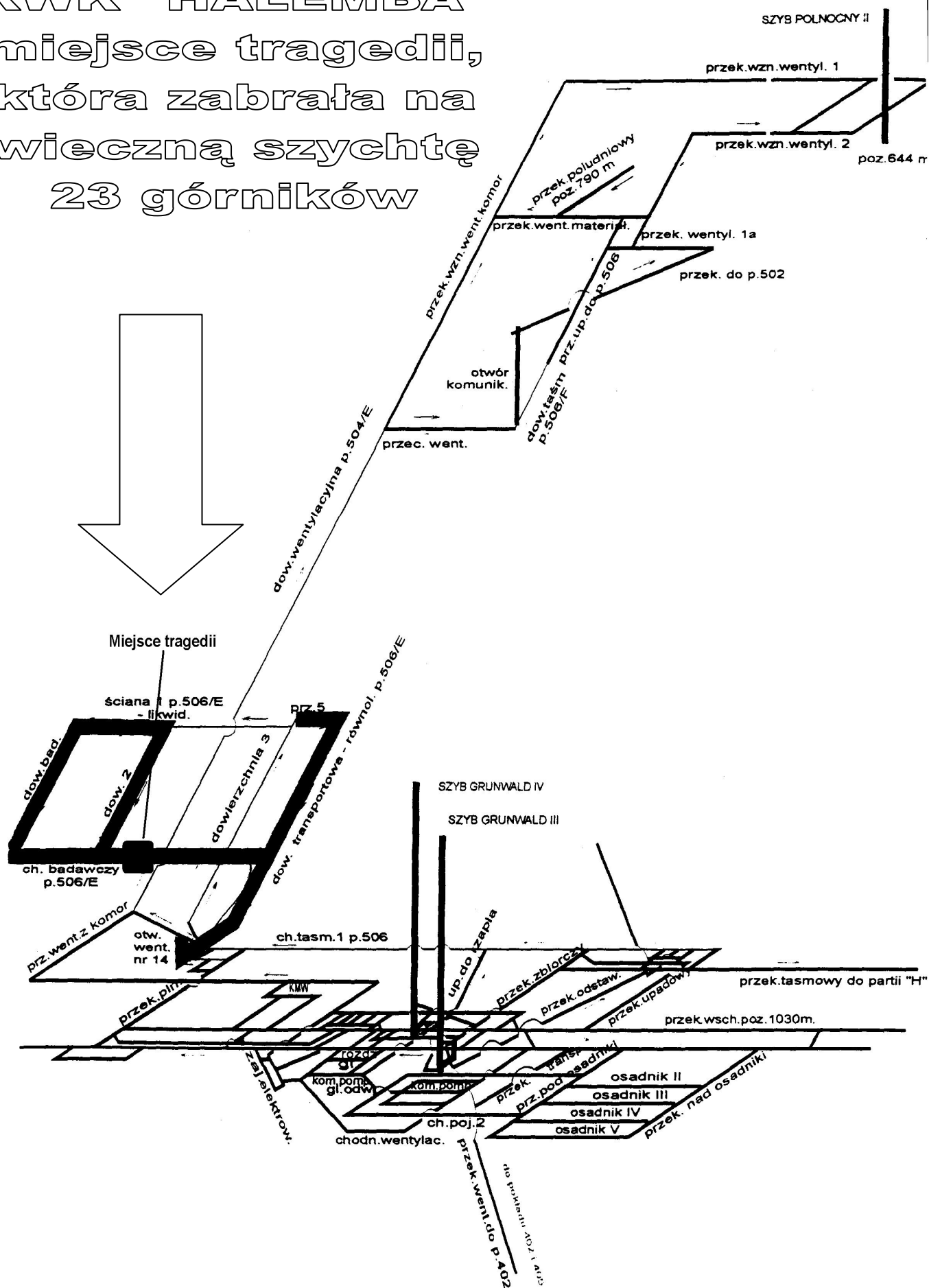
Rys.6. Wyrobiska w pokł. 506/E w których zostały przekroczone parametry klimatyczne
